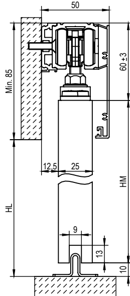
Wandmontage mit Abstandsprofil sliding door at wall with spacer
