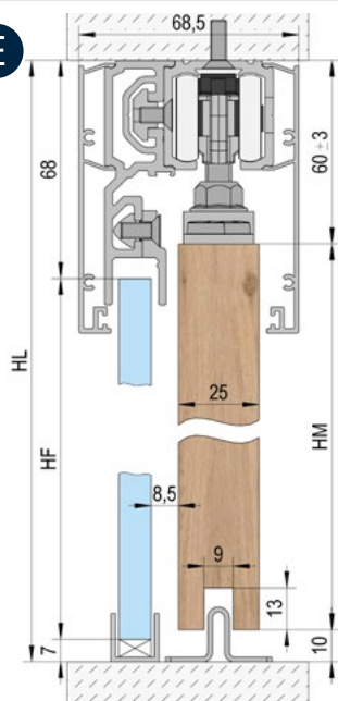
Montage au plafond / 1 vantail / avec vitrage fix
