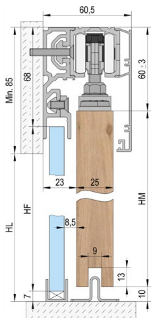
Montage mural / 1 vantail / avec vitrage fixe
