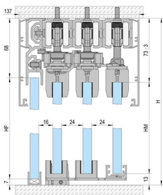
Montage plafond / 3 vantaux / avec pan fixe
