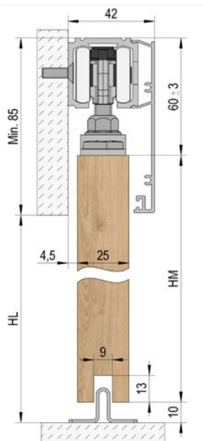
Montage mural / 1 vantail
