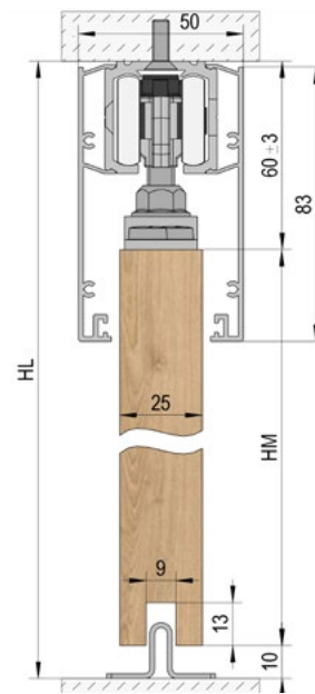
Montage au plafond / 1 vantail
