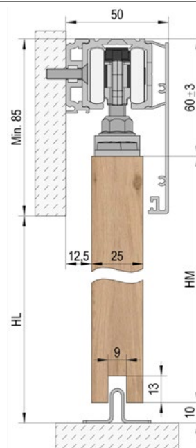
Montage mural / 1 vantail / avec profilé d'écartement mural
