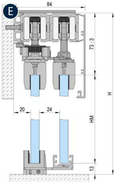
Falra szerelés / 2 szárnyú
