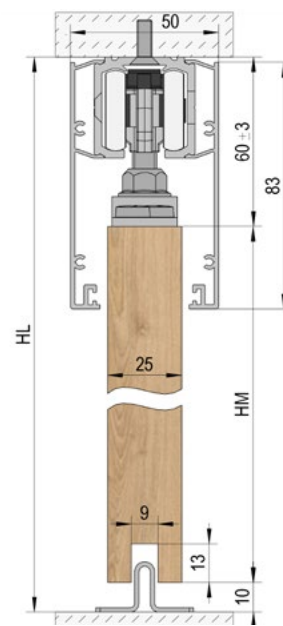
Mennyezeti szerelés / 1 szárnyú
