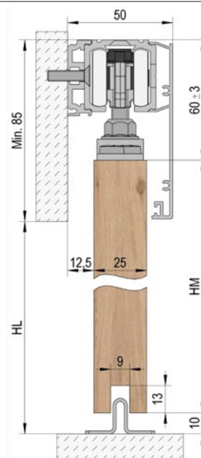
Falra szerelhető / 1 szárnyú / fali távtartó profillal
