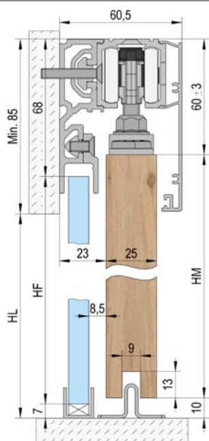
Falra szerelhető / 1 szárnyú / fix üvegezéssel
