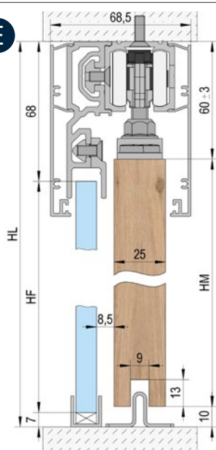
Mennyezeti szerelés / 1 szárnyú / fix üvegezéssel
