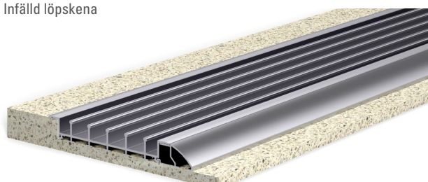
Infälld löpskena med en rampprofil
