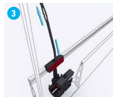
Schritt 3 - Verankern
