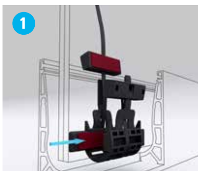
Schritt 1 - Fixieren
