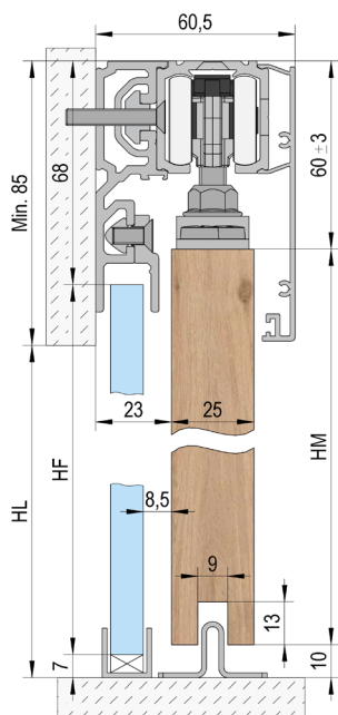
Montaggio a parete / a 1 anta / con vetro fisso
