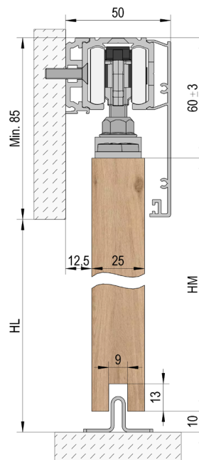
Montaggio a parete / a 1 anta / con profilo distanziatore a parete
