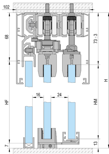
Plafondinbouw / 2-vleugelig / met vaste beglazing
