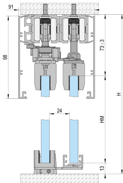
Plafondinbouw / 2-vleugelig
