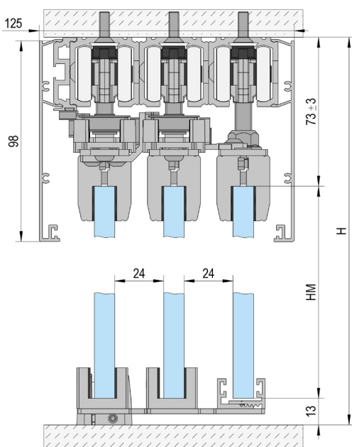
Plafondinbouw / 3-vleugelig
