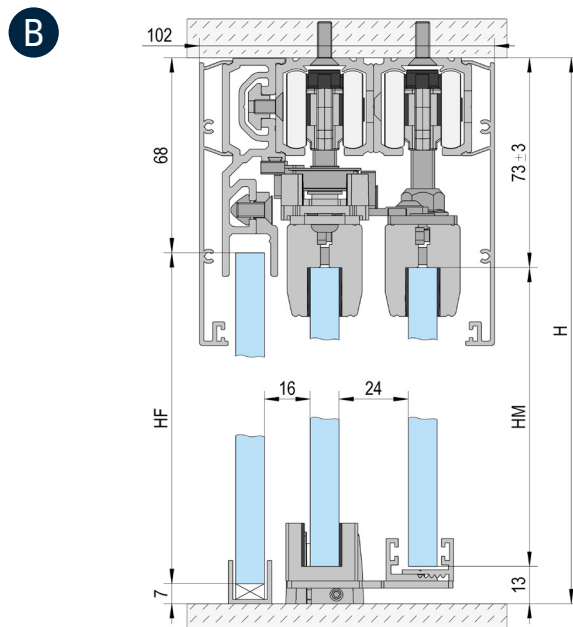
Montaje en el techo / 2 hojas / con acristalamiento fijo
