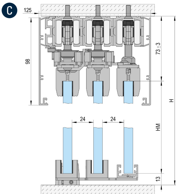
Montaje en el techo / 3 hojas
