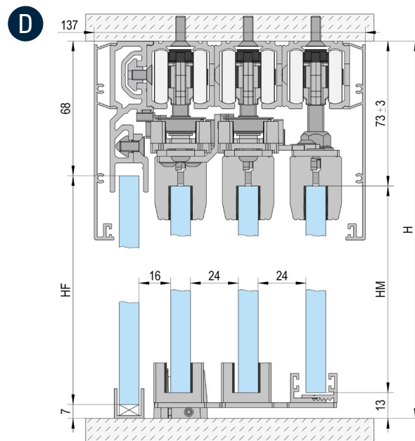
Montaje en el techo / 3 hojas / con acristalamiento fijo
