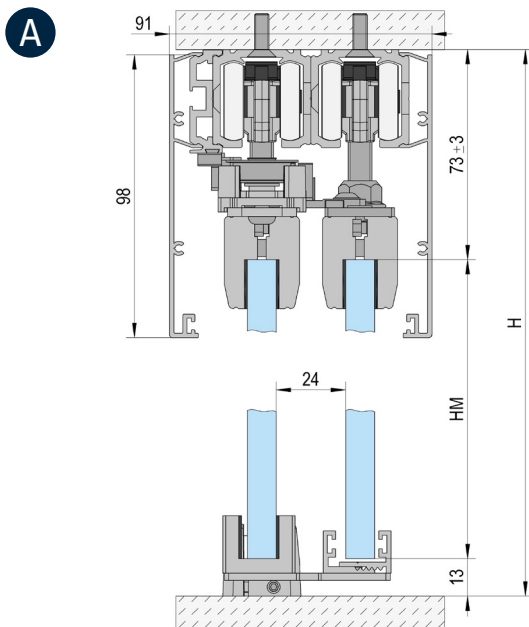
Montaje en el techo / 2 hojas
