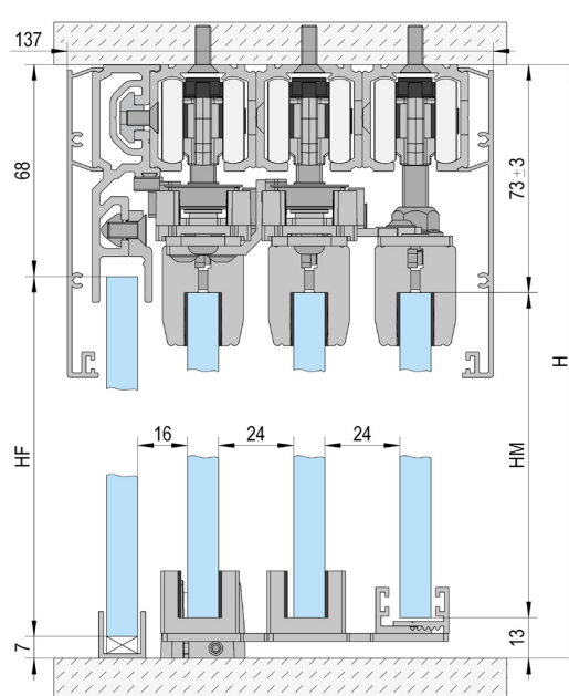
Mennyezetre szerelés / 3 szárnyú / fix-üvegezéssel
