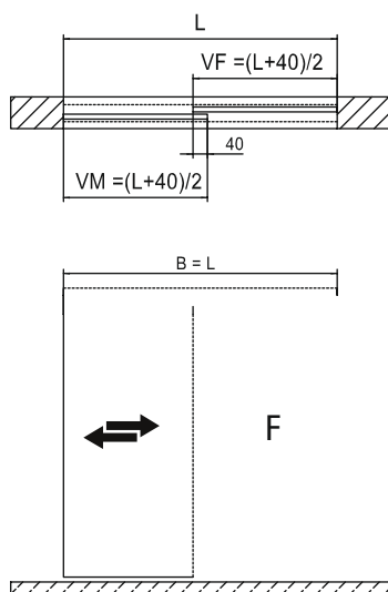
Eine Schiebetür Deckenmontage mit Festverglasung / Wandtasche 1 sliding door + 1 fixed glass - wall recess
