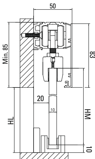
Wandmontage mit Abstandsprofil sliding door at wall with spacer
